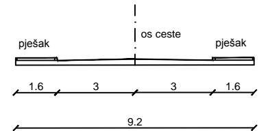
KARAKTERISTIČAN POPREČNI PRESJEK C-C MJ. 1:200
