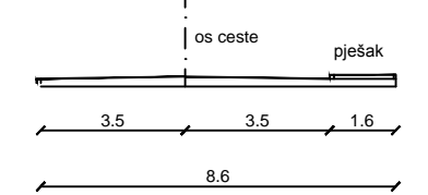
KARAKTERISTIČAN POPREČNI PRESJEK C-C MJ. 1:200
