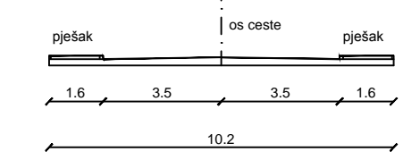
KARAKTERISTIČAN POPREČNI PRESJEK B-B MJ. 1:200
