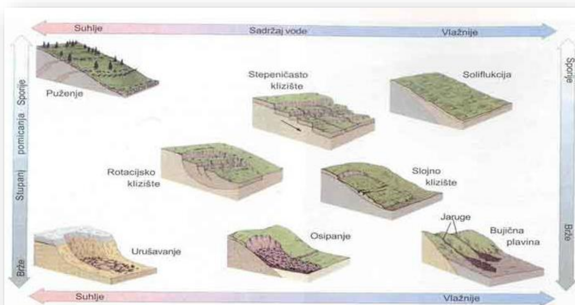
Vrste klizišta
